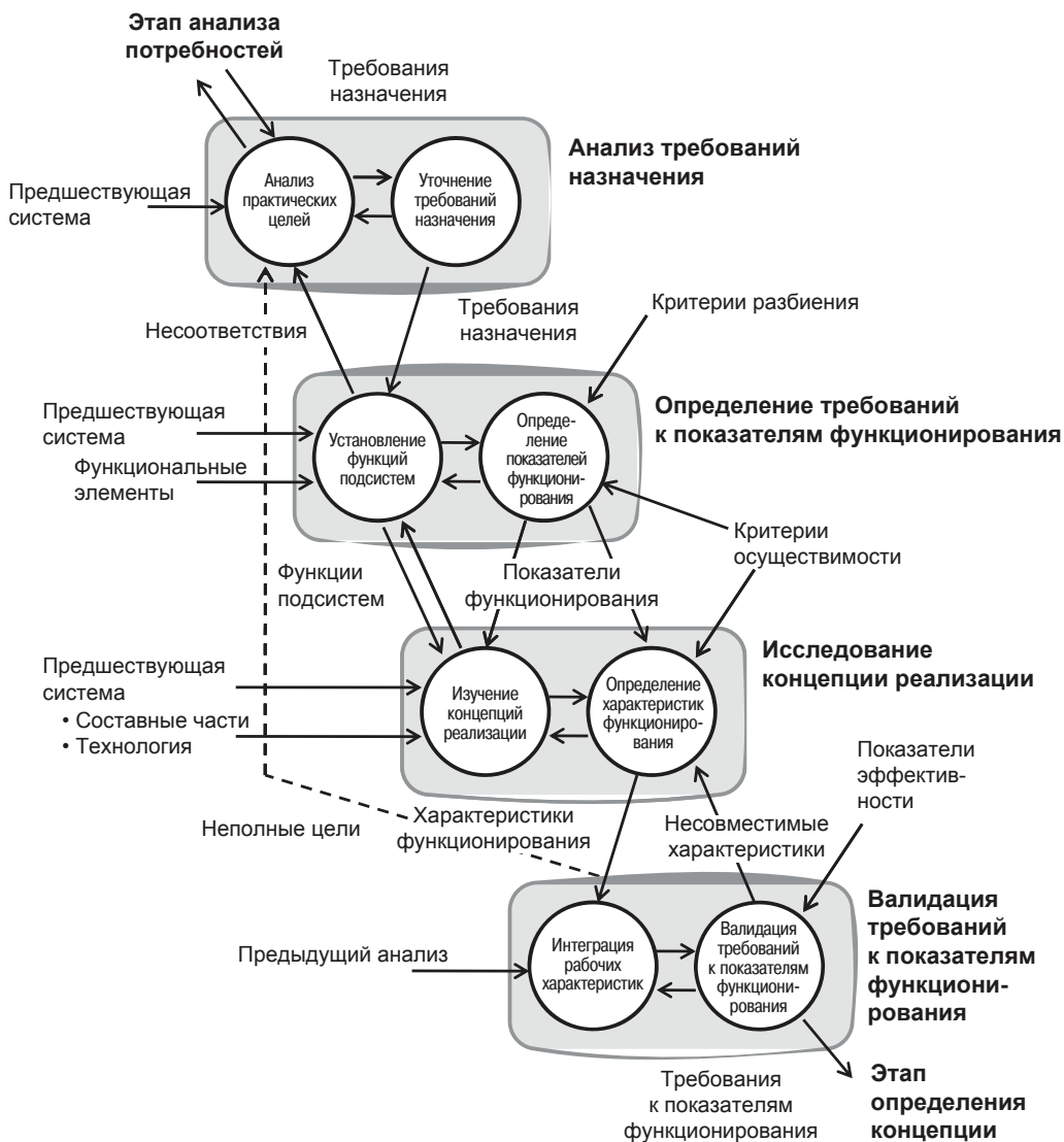
Рис. 7.2. Блок-схема этапа исследования концепции
