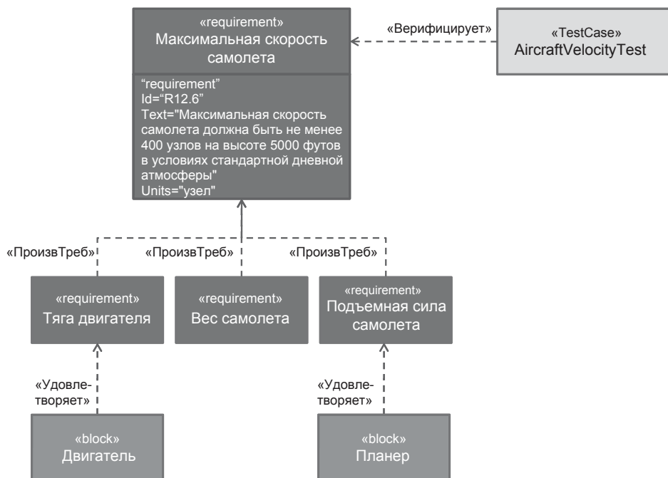
Рис. 8.15. Диаграмма требований в SysML
