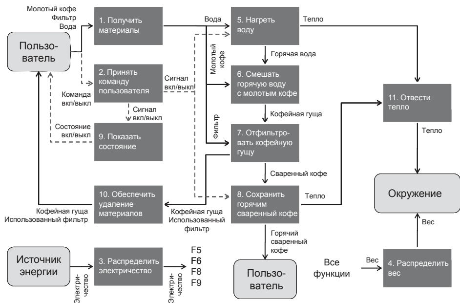
Рис. 8.4. Функциональная блок-схема стандартной кофеварки
