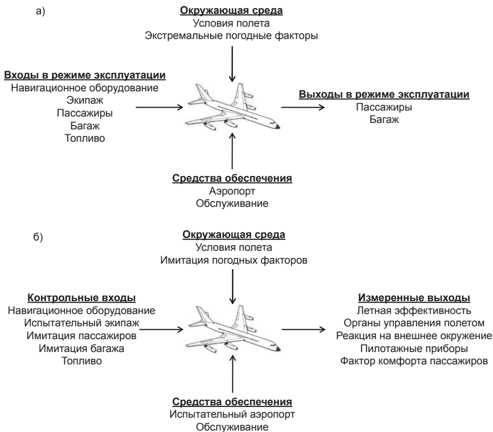
Рис. 13.6: а) функционирование пассажирского авиалайнера; б) натурные испытания авиалайнера
