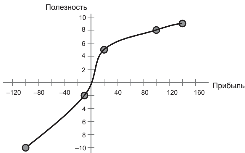
Рис. 9.17. Функция полезности
