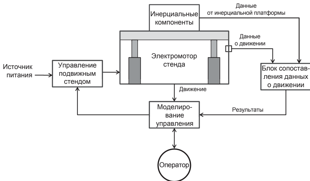
Рис. 9.6. Программно-аппаратная модель
