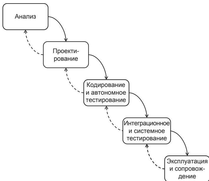
Рис. 11.4. Классическая каскадная модель жизненного цикла разработки ПО
