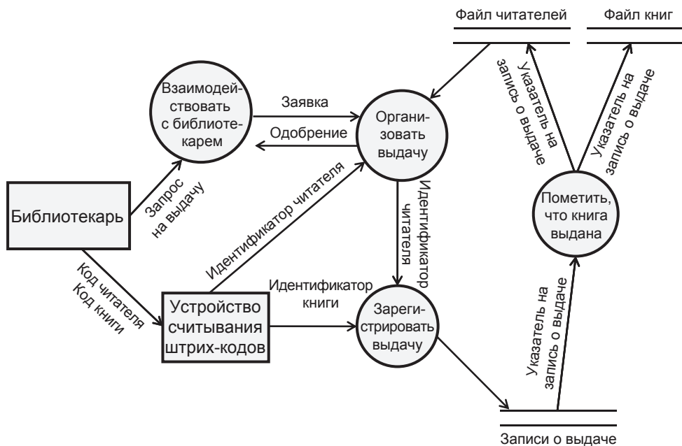
Рис. 11.12. Диаграмма потоков данных: выдача книги из библиотеки
