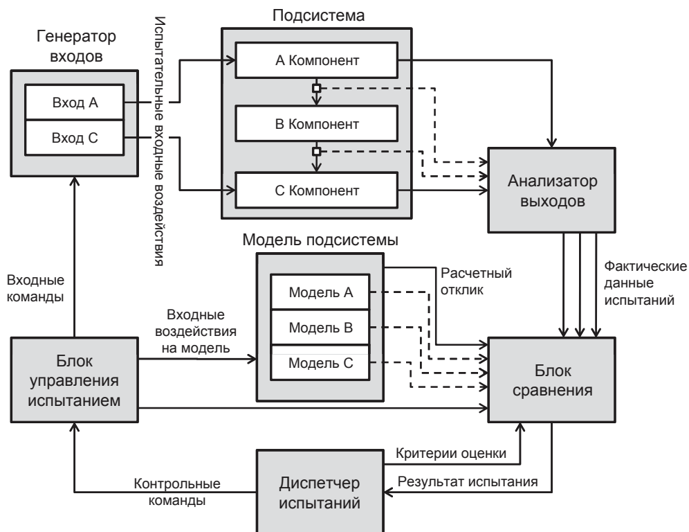
Рис. 13.5. Схема установки для испытания элемента системы
