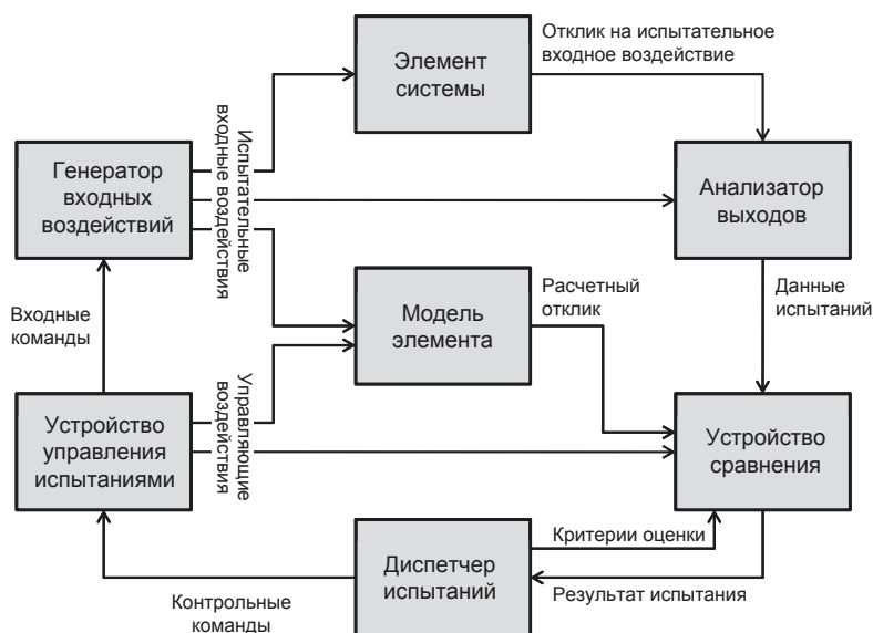
Рис. 13.4. Схема установки для испытания элемента системы
