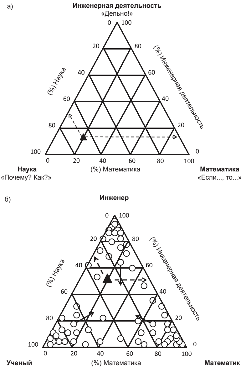
Рис. 1.2. а) Техническая ориентация. Фазовая диаграмма. б) Техническая ориентация. Распределение плотности
