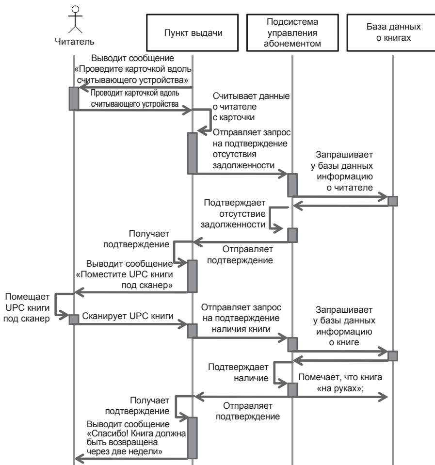
Рис. 8.10. UML-диаграмма последовательности
