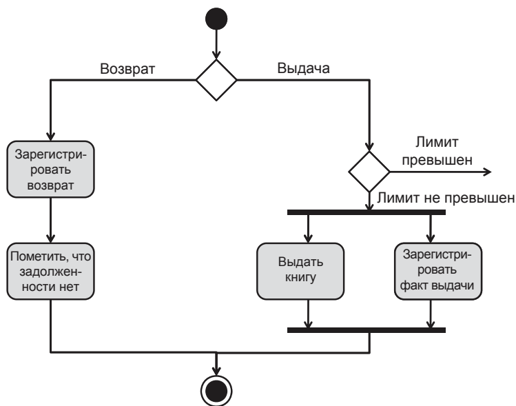
Рис. 8.9. UML-диаграмма деятельности
