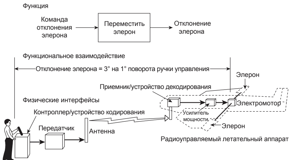
Рис. 3.5. Функциональные взаимодействия и физические интерфейсы
